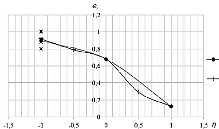
Рис. 4. Діаграма пластичності сплаву W-Ni-Fe[2].
