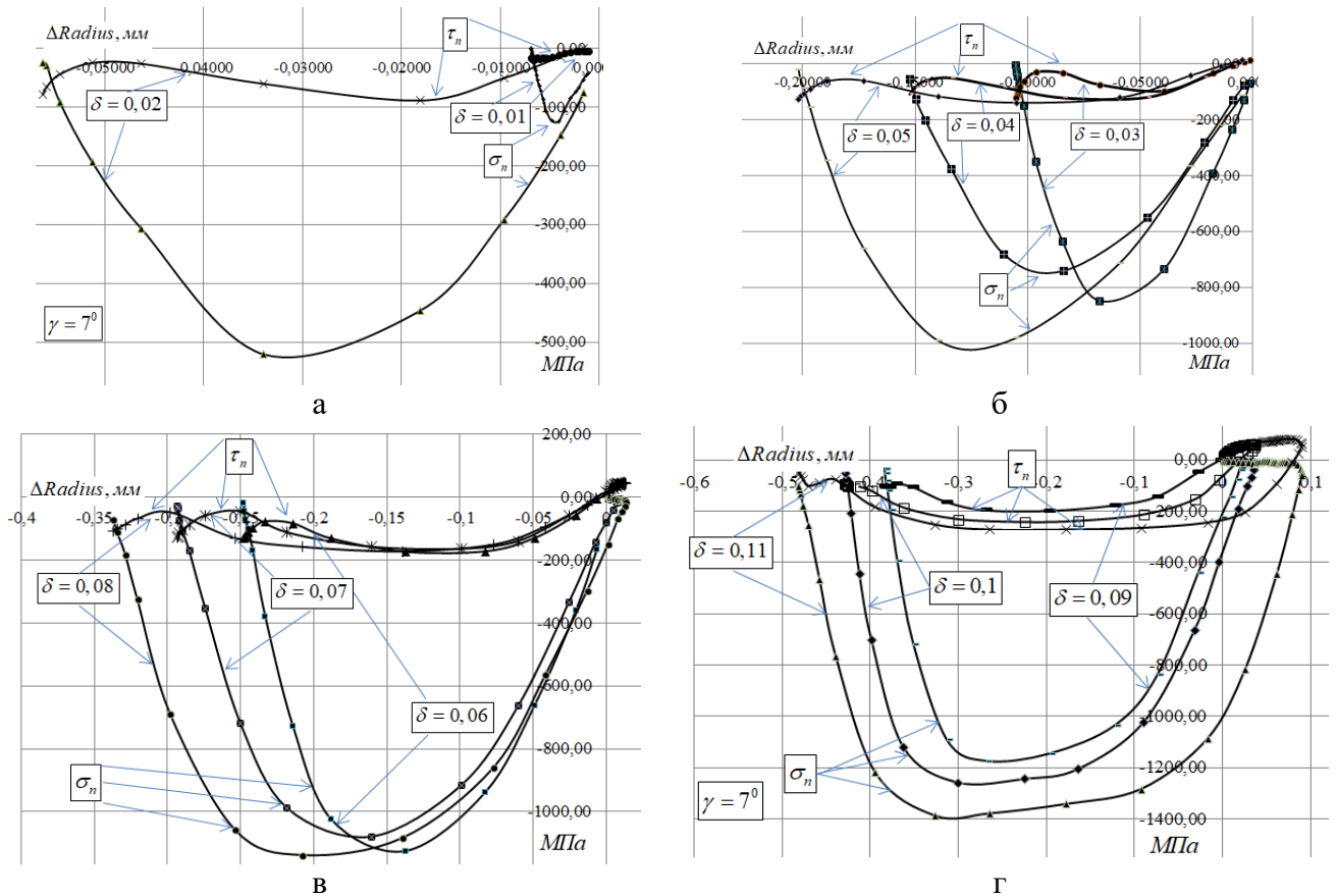
Рис. 5. Значення контактних напружень по контуру матриці для процесу редукування з кутом нахилу матриці \gamma = 7^\circ та різних обтисків ( \delta = 0,01; 0,02; 0,03; 0,04; 0,05; 0,06; 0,07; 0,08; 0,09; 0,1; 0,11 )
