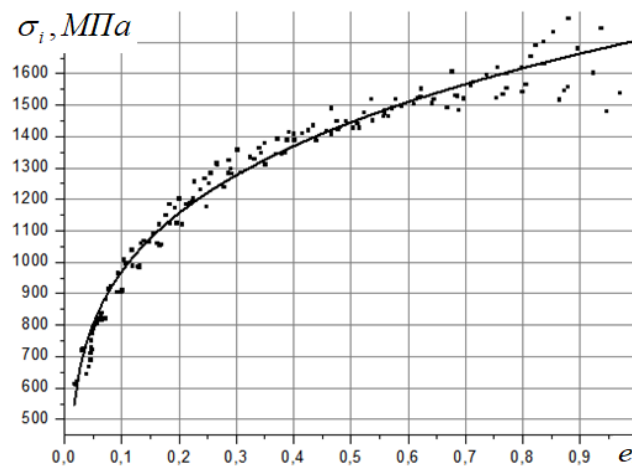
Рис. 3. Крива течії сплаву W-Ni-Fe.
