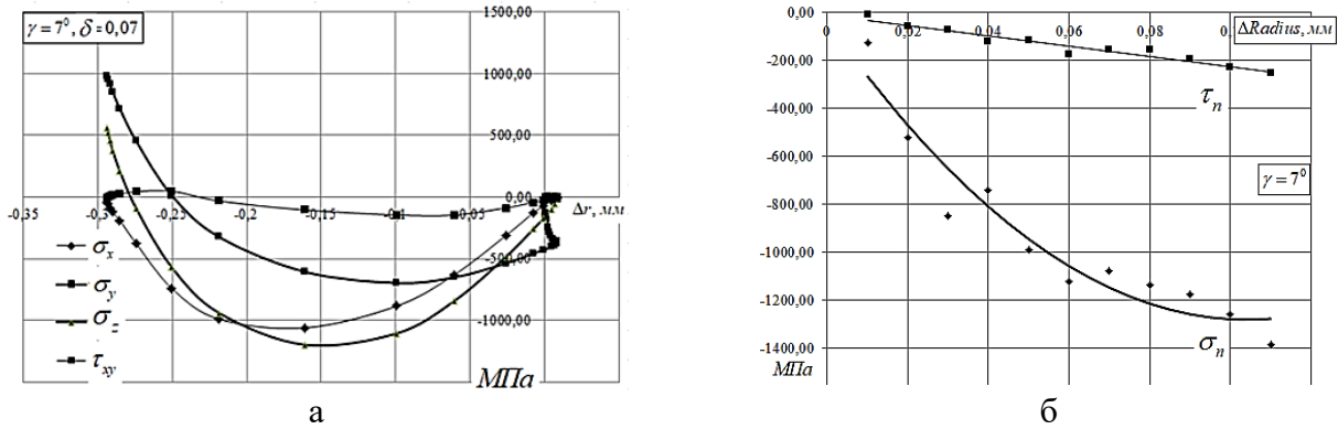
Рис. 6. Зміна величини компонент тензора напружень \sigma_z , \sigma_r , \sigma_\varphi , \tau_{rz} в контактній області (а) та значення максимальних контактних напружень по контуру матриці для процесу редукування з кутом нахилу матриці \gamma = 7^\circ (б)
