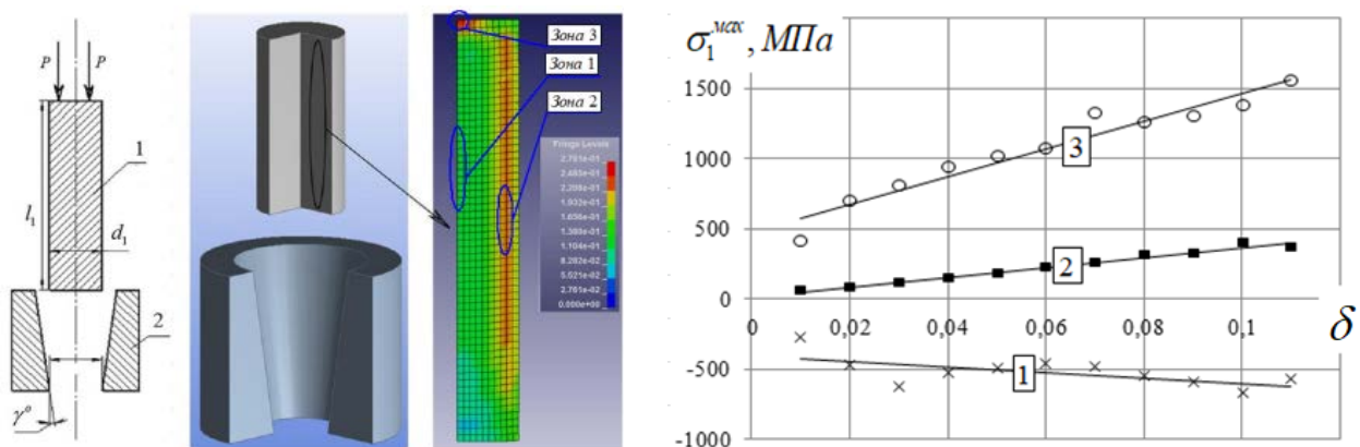
Рис. 1. Залежність максимальних головних нормальних напружень від величини відносного обтиску
